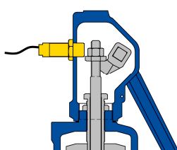
Type avec détecteur d'activation
