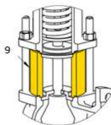
Type avec insert 614, 674
