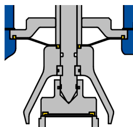
Type avec membrane (01-4)
