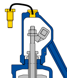
Type avec vis de verrouillage (test gag)
