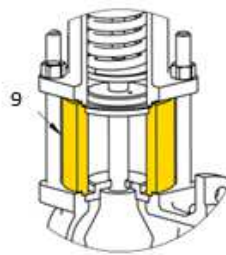
Type avec insert 613, 673
